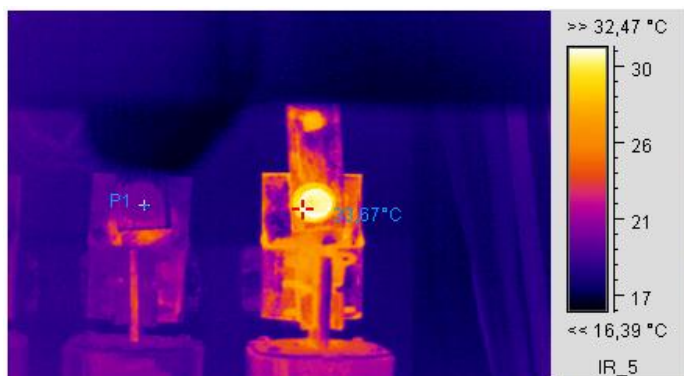
Термограмма 1
