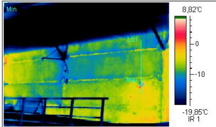
Термограмма 2
