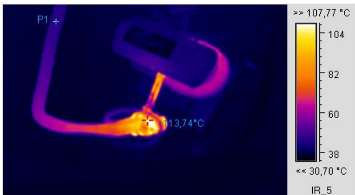
Термограмма 1
