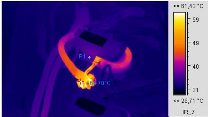
Термограмма 2
