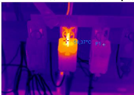
Термограмма 4
