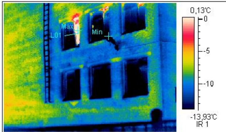
Термограмма 6
