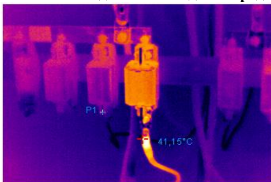
Термограмма 2
