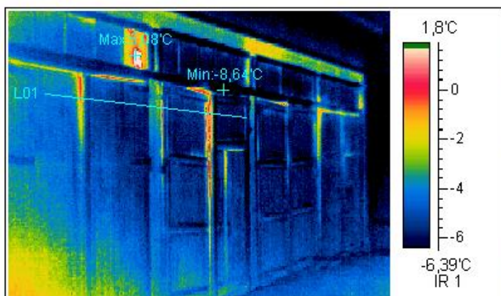
Термограмма 1
