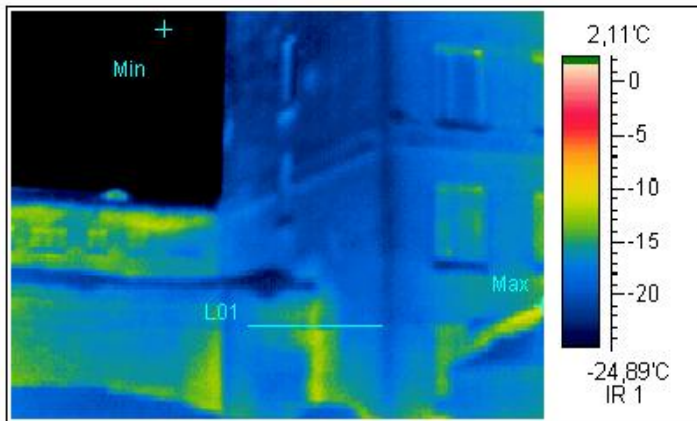
Термограмма 7
