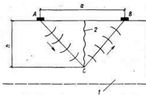
Рис. 1. Определение глубины поверхностной трещины в бетоне
