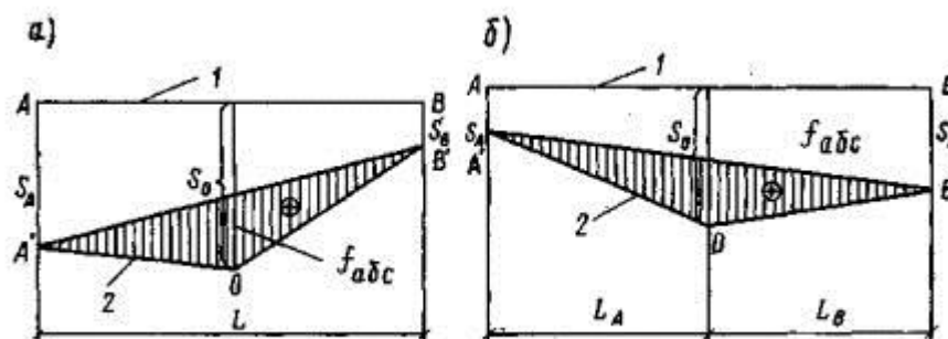
Рис. 4. Схема определения прогиба фундамента
