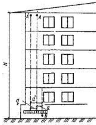
Рис. 5. Схема измерений крена зданий:
