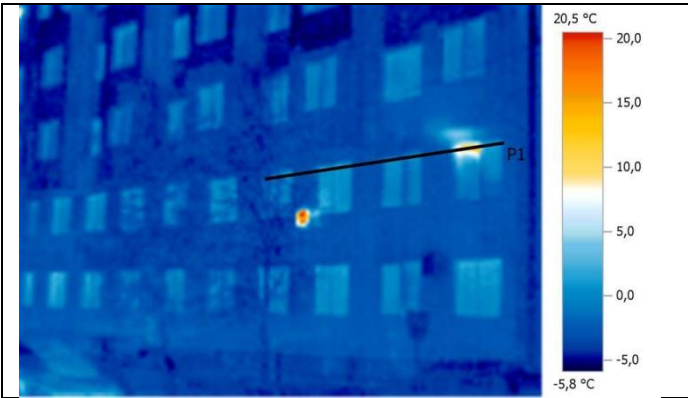
Термограмма №8
