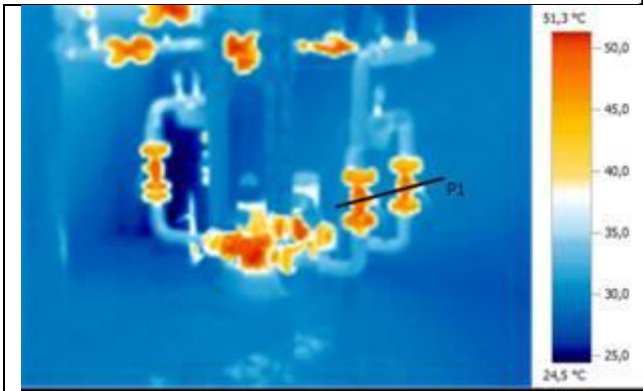
Термограмма №1
