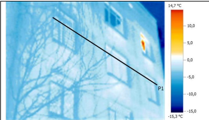
Термограмма №3
