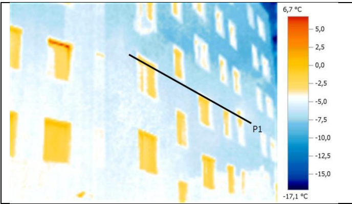
Термограмма №9
