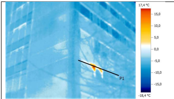
Термограмма №14
