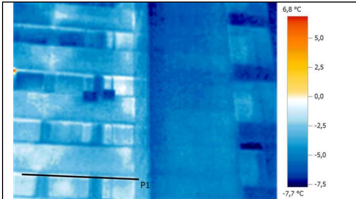
Термограмма №13
