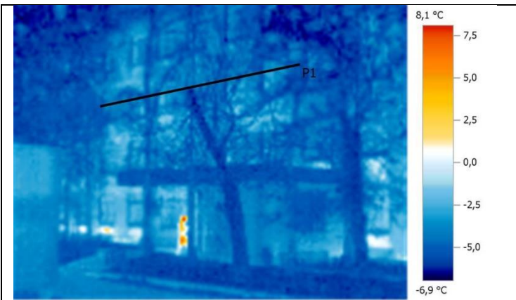
Термограмма №2
