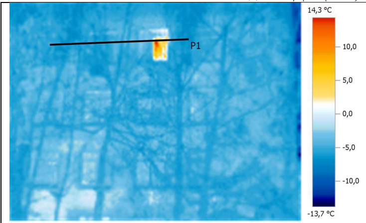
Термограмма №1
