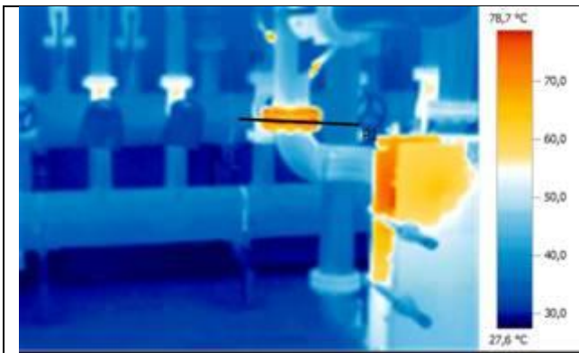
Термограмма №2
