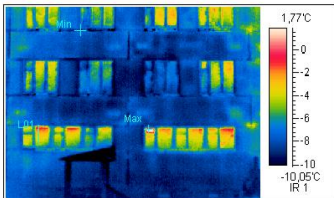
Термограмма 5
