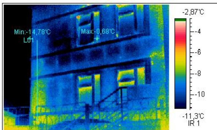
Термограмма 5
