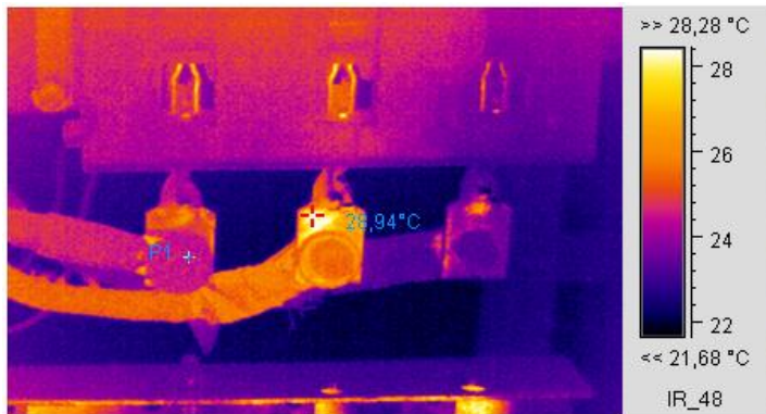
Термограмма 1
