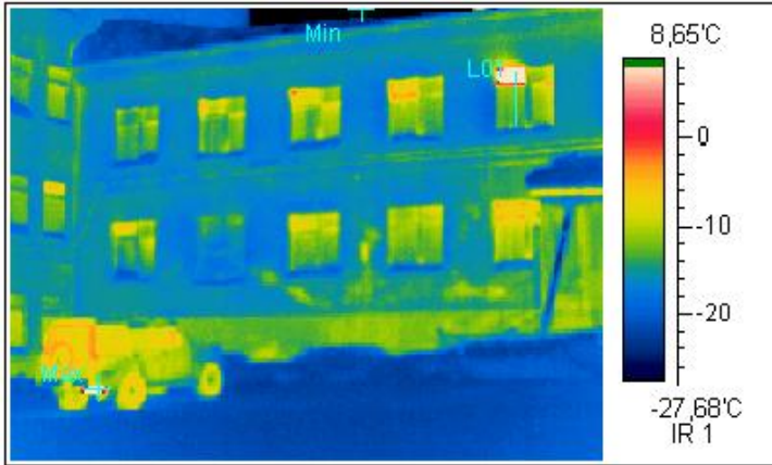
Термограмма 1
