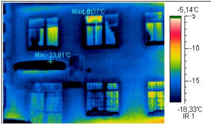
Термограмма 6
