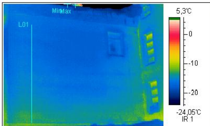
Термограмма 5
