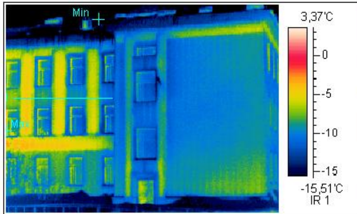
Термограмма 2
