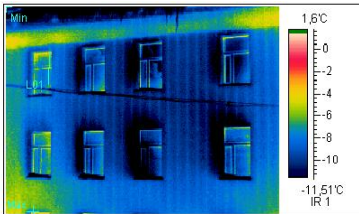
Термограмма 3
