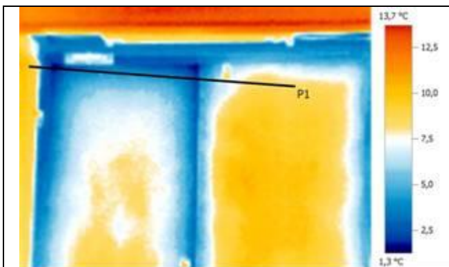
Дверной проем. Сторона А-Б.
