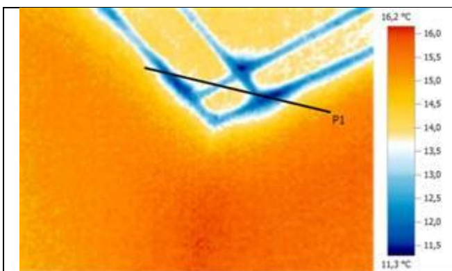
Угловой стык. Кабинет. Угол Б-2.
