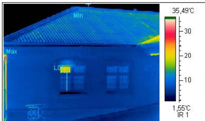
Термограмма 1
