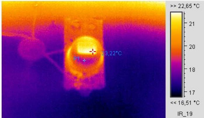
Термограмма 1
