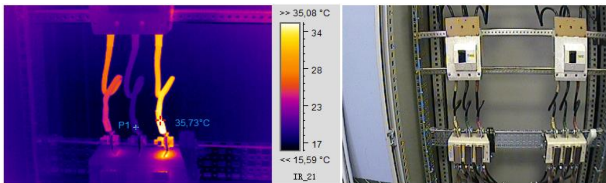
Термограмма 5
