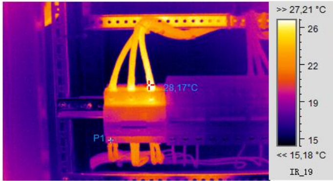
Термограмма 4
