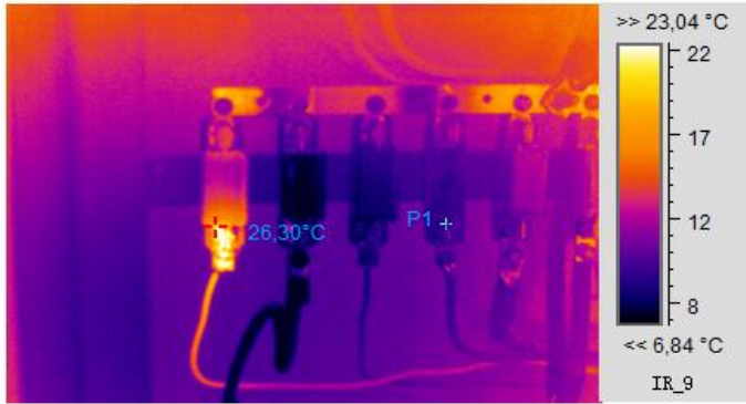
Термограмма 4
