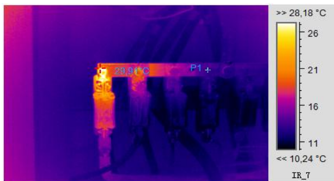
Термограмма 3
