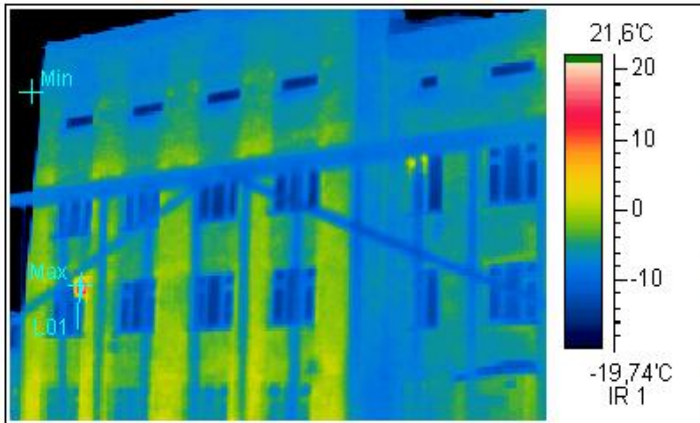
Термограмма 7
