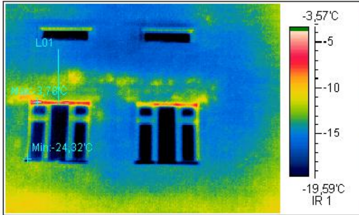
Термограмма 5
