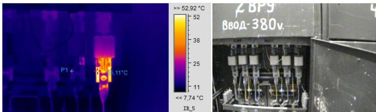
Термограмма 2
