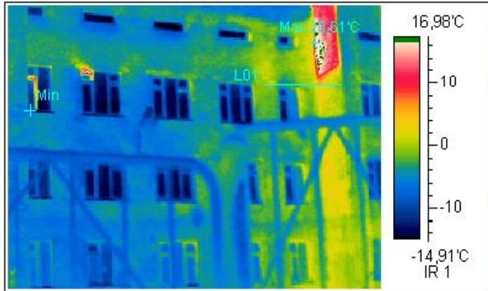
Термограмма 8
