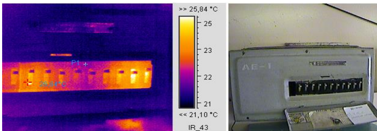
Термограмма 1
