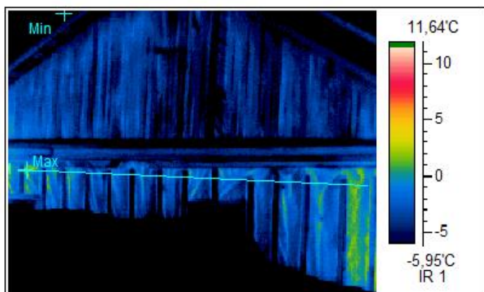
Термограмма 2
