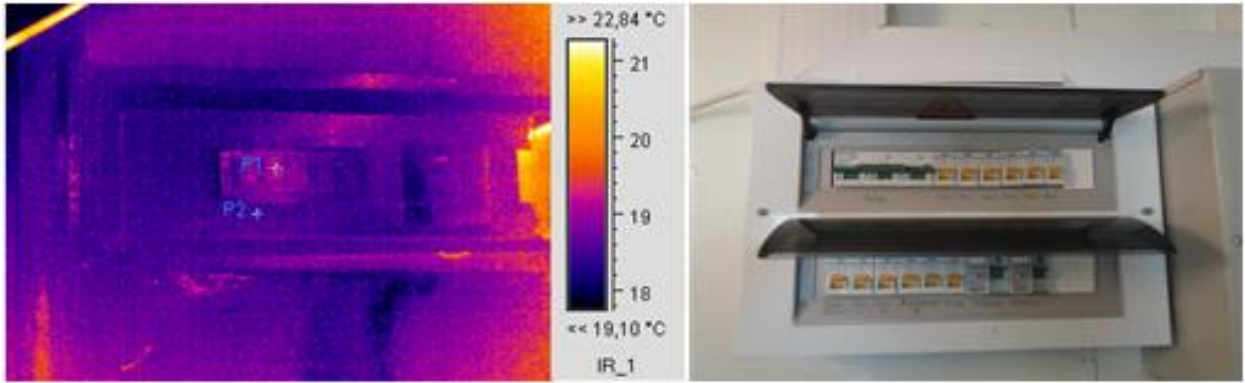
Термограмма 1
