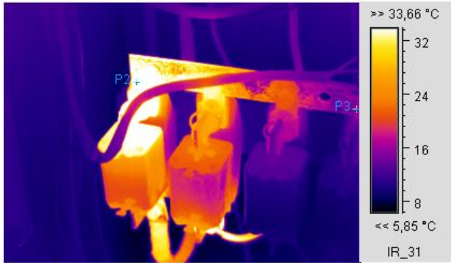
Термограмма 4
