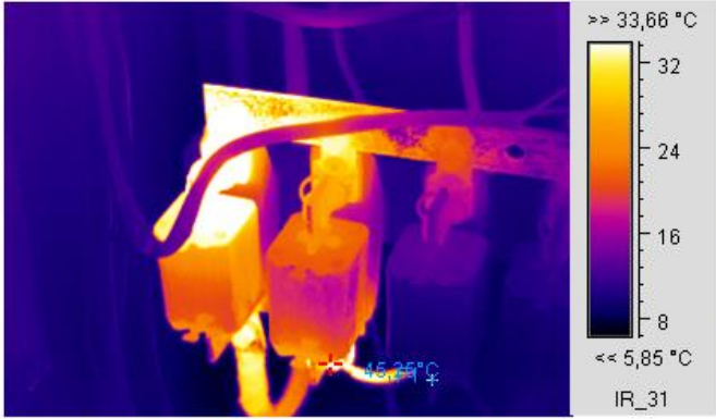
Термограмма 3
