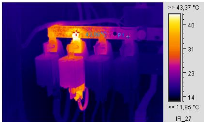
Термограмма 1
