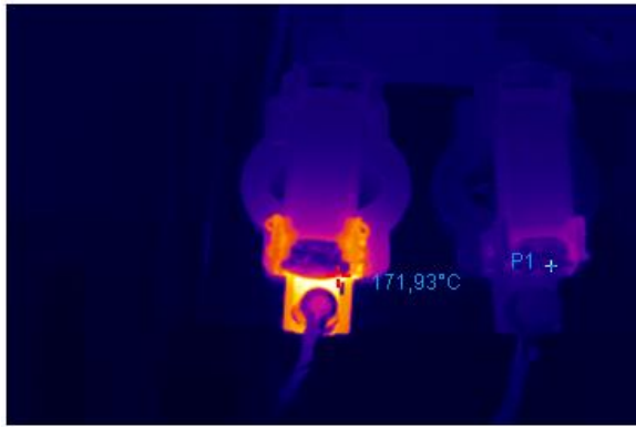
Термограмма 2
