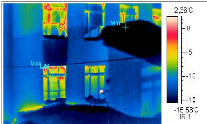
Термограмма 3
