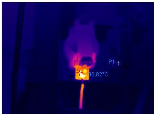
Термограмма 1
