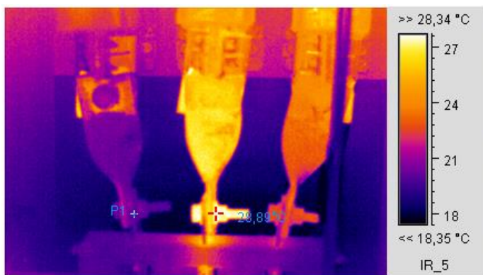
Термограмма 3
