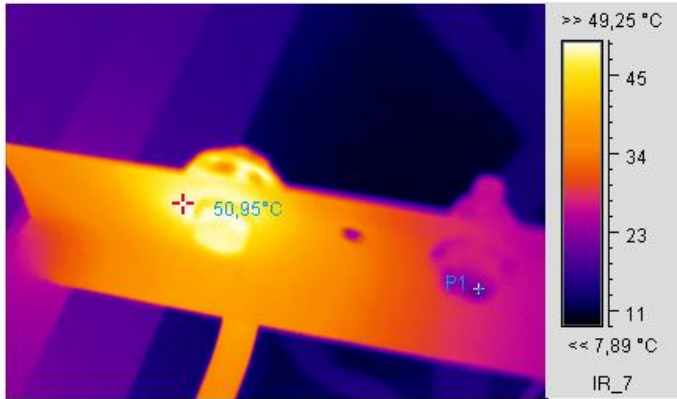
Термограмма 4
