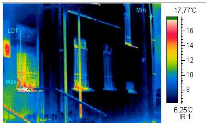
Термограмма 6
