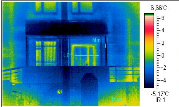
Термограмма 5
