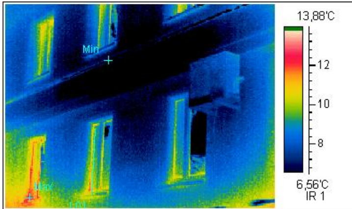
Термограмма 2
