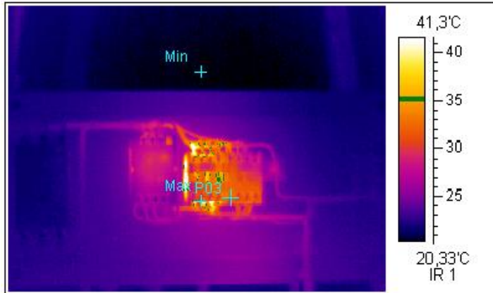
Термограмма 7
