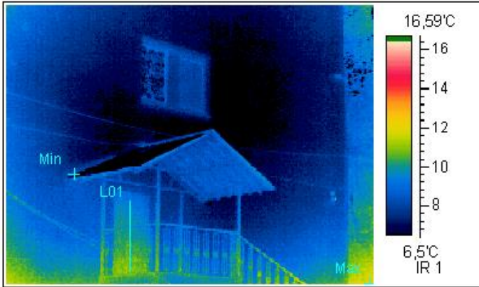
Термограмма 6
