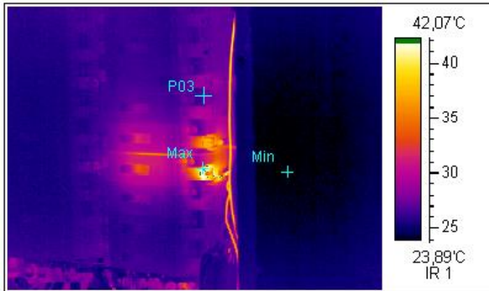
Термограмма 8
