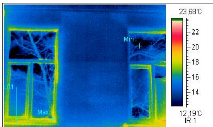
Термограмма 2
