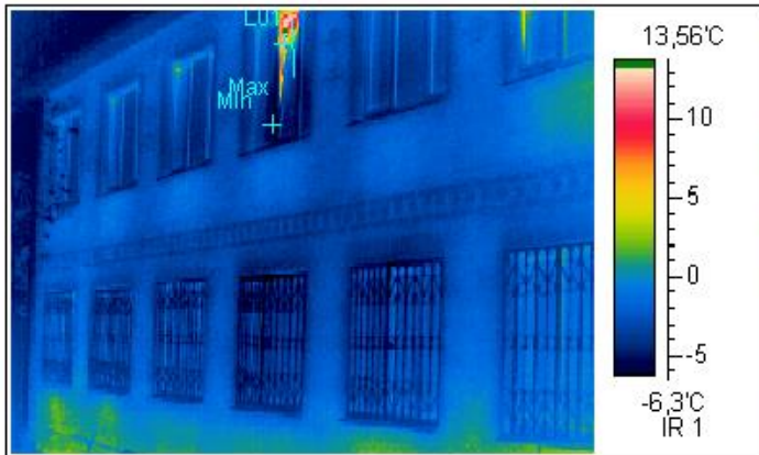
Термограмма 5
