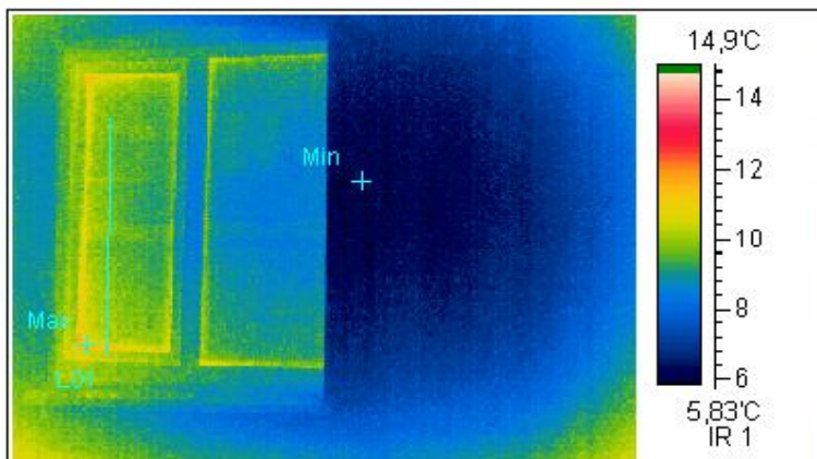
Термограмма 3
