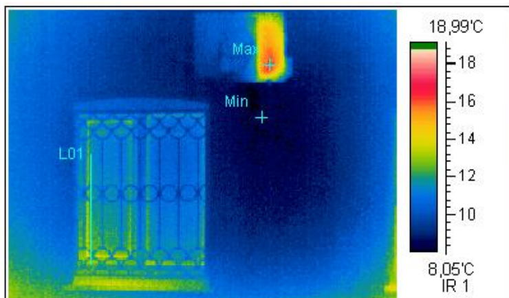
Термограмма 1
