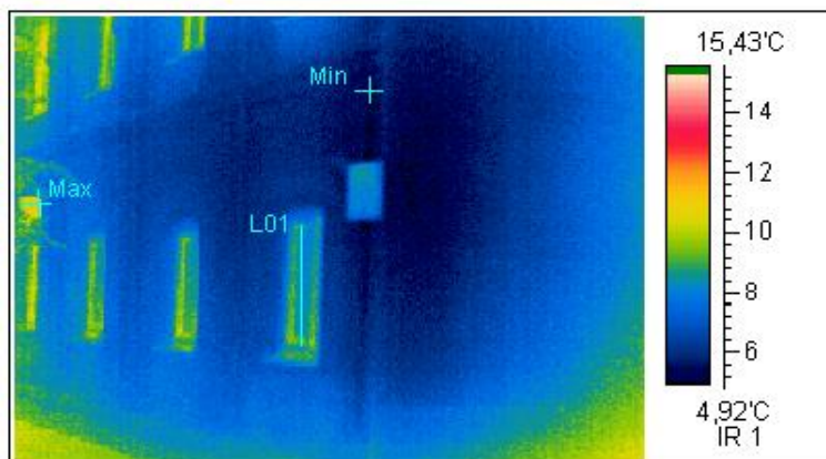
Термограмма 4
