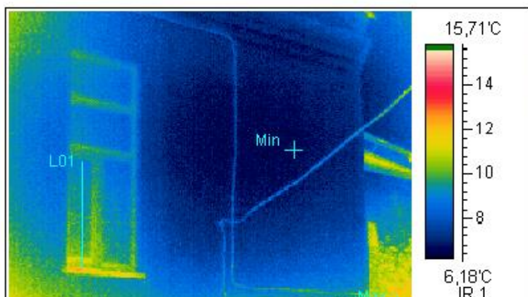
Термограмма 2
