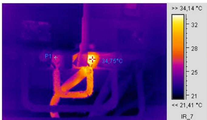
Термограмма 2
