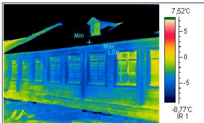
Термограмма 5
