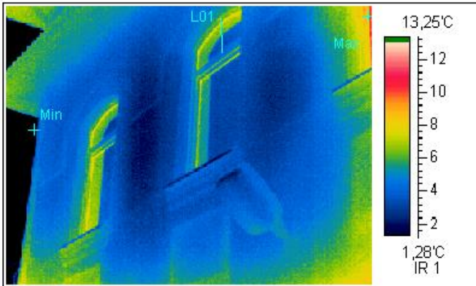
Термограмма 5
