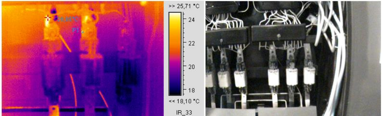
Термограмма 1
