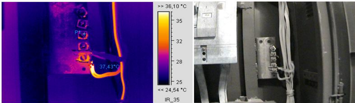
Термограмма 2
