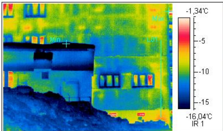
Термограмма 2
