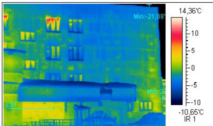
Термограмма 1
