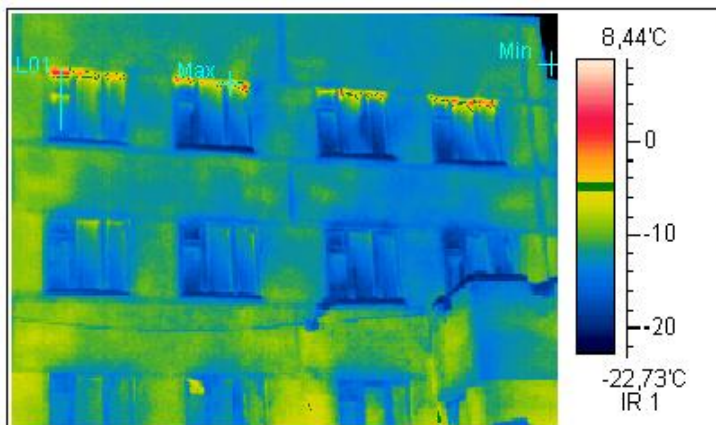
Термограмма 8
