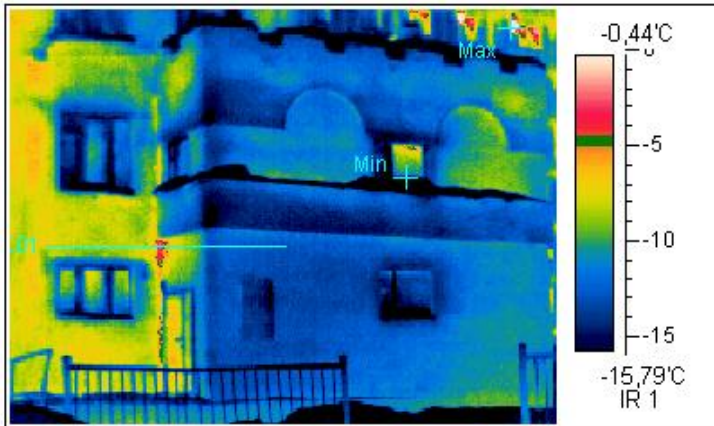
Термограмма 7
