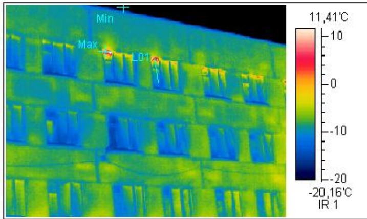
Термограмма 6
