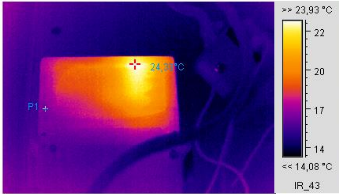
Термограмма 1
