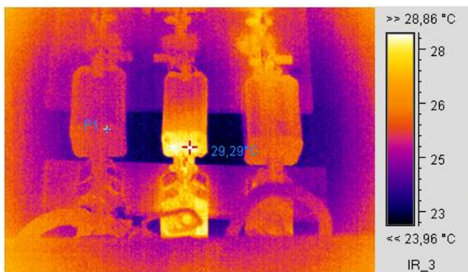
Термограмма 2
