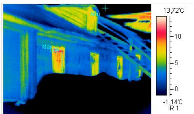
Термограмма 7
