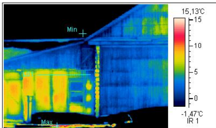
Термограмма 2
