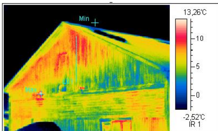
Термограмма 9
