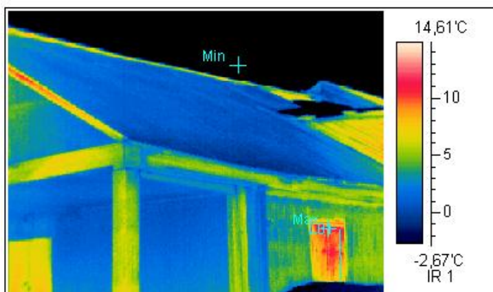
Термограмма 4
