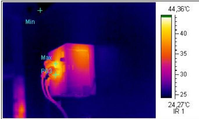
Термограмма 4
