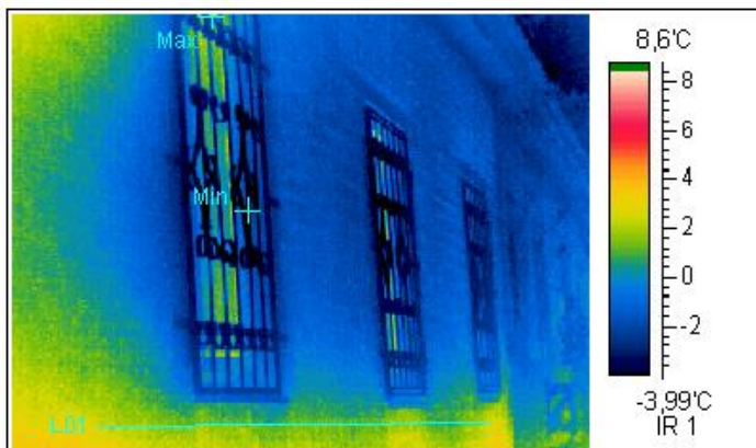
Термограмма 12
