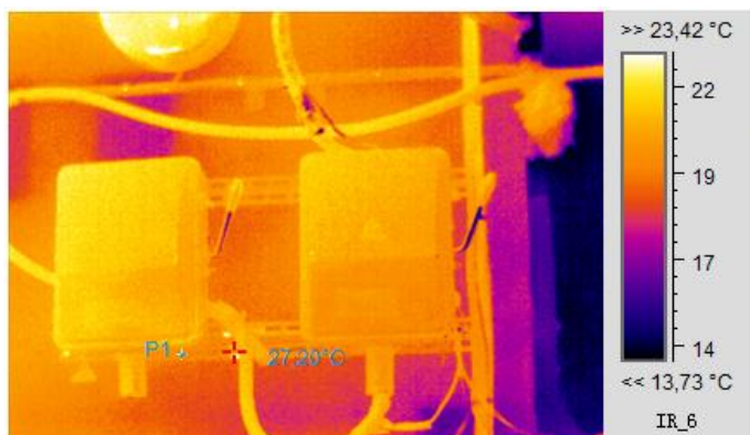
Термограмма 1
