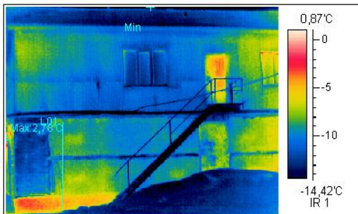
Термограмма 12
