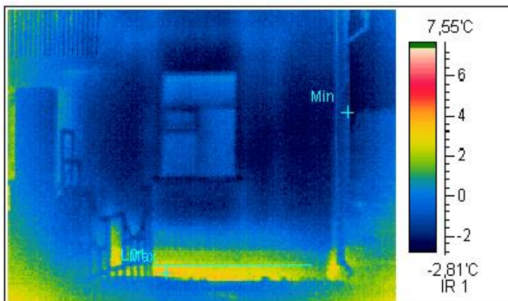
Термограмма 5
