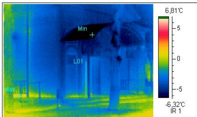
Термограмма 4
