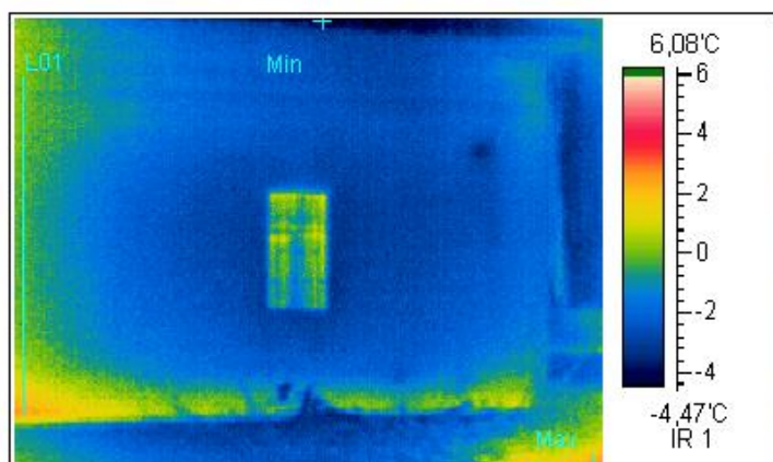
Термограмма 1
