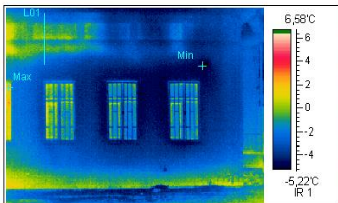
Термограмма 3
