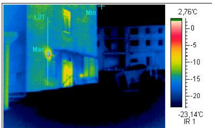
Термограмма 3
