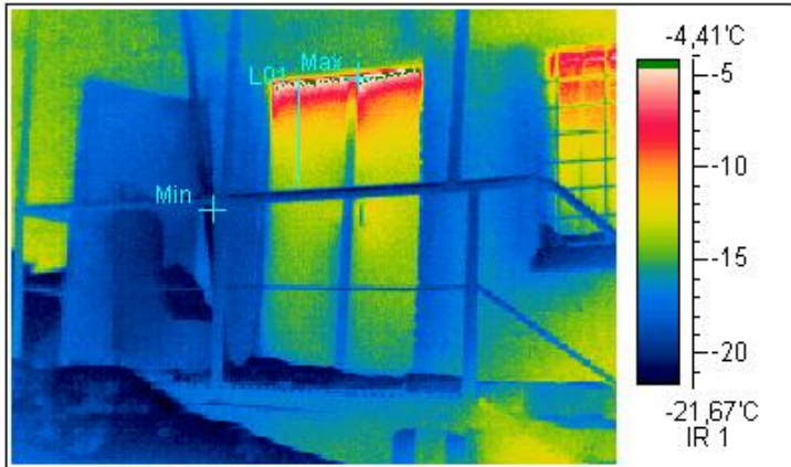
Термограмма 6
