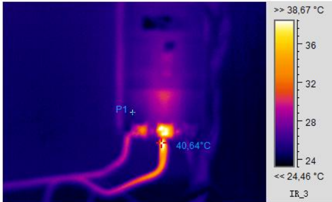
Термограмма 1
