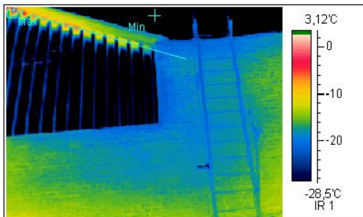
Термограмма 8
