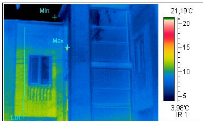
Термограмма 4
