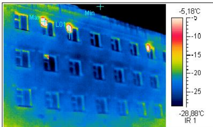
Термограмма 3
