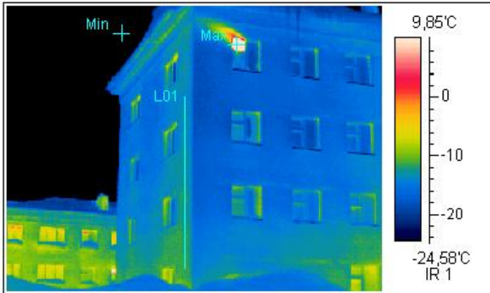
Термограмма 7
