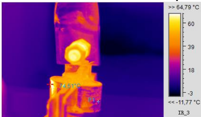
Термограмма 2
