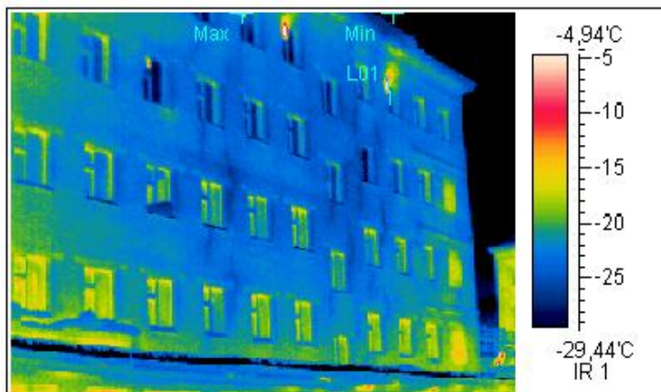
Термограмма 5
