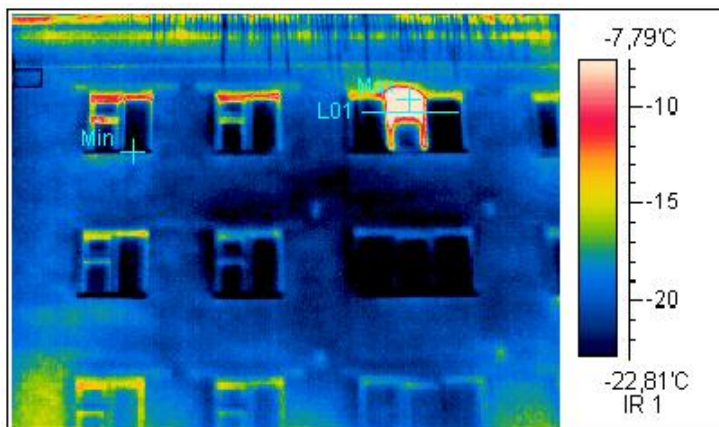
Термограмма 2
