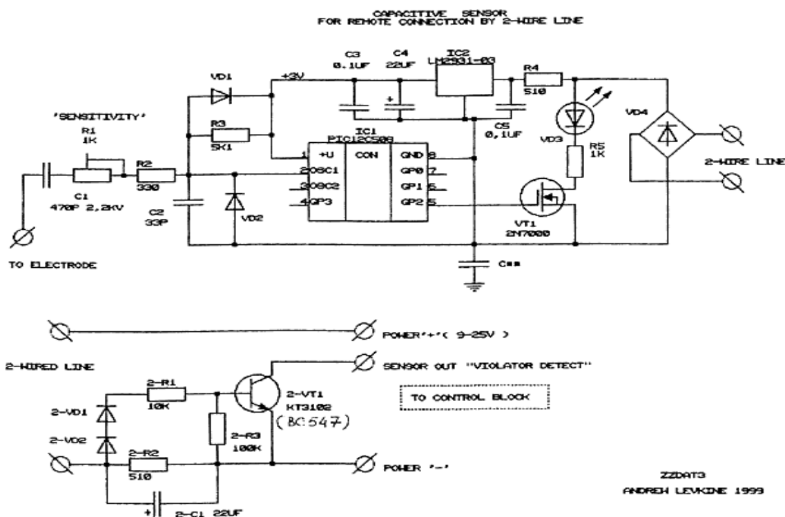
Рис. 4.1 Принципиальная микросхема датчика движения-присутствия «Контроль-Люкс 180°»
