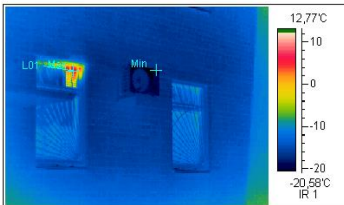
Термограмма 5
