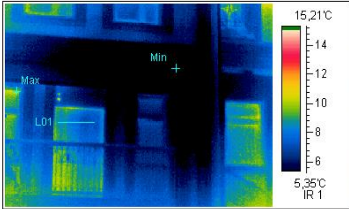
Термограмма 2
