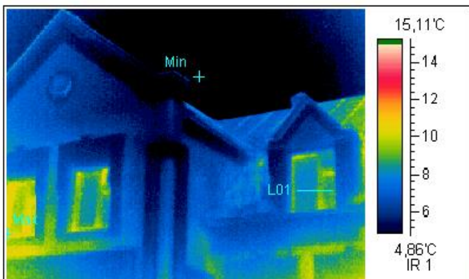
Термограмма 3
