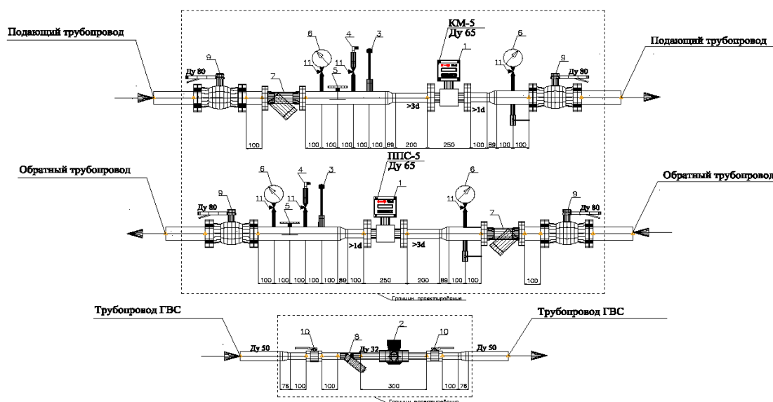
Рис.2 Принципиальная схема системы учета теплопотребления
