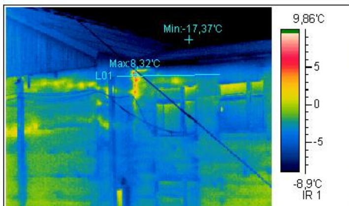
Термограмма 6
