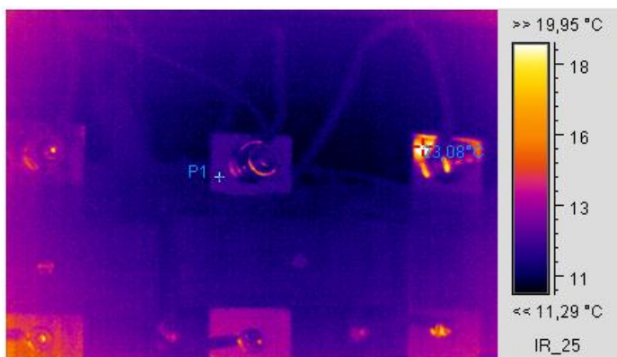
Термограмма 2
