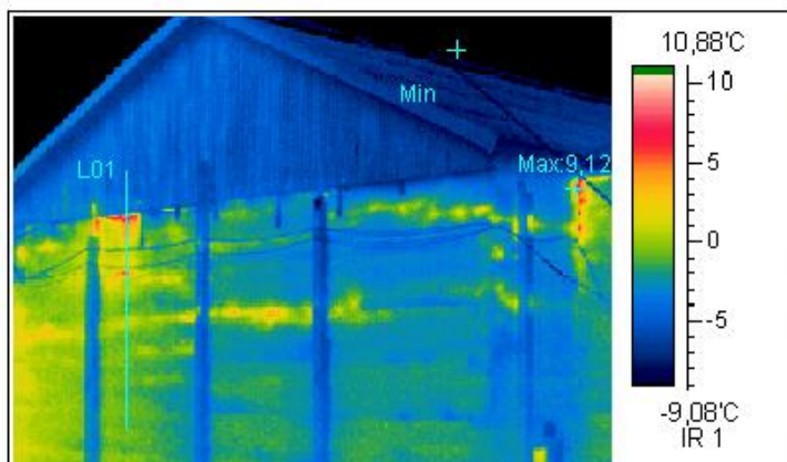
Термограмма 5
