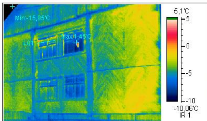
Термограмма 3
