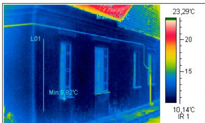
Термограмма 4
