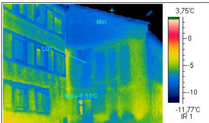
Термограмма 6
