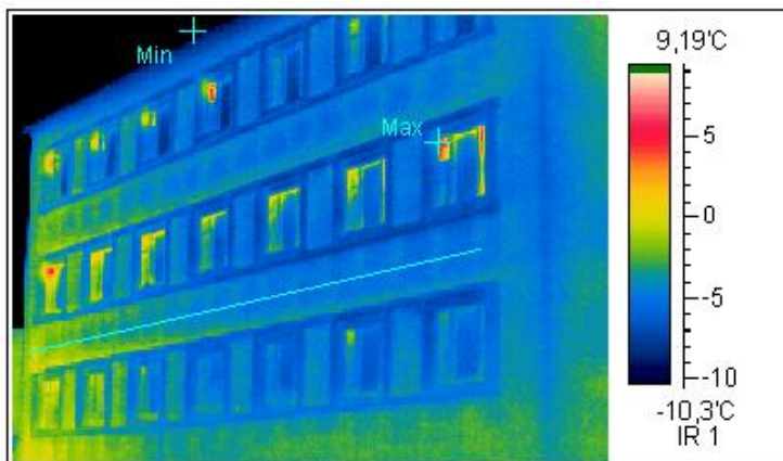
Термограмма 5
