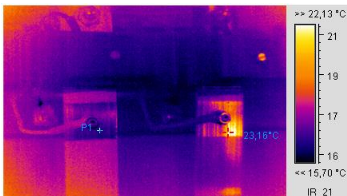
Термограмма 2
