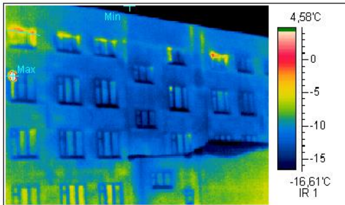
Термограмма 6
