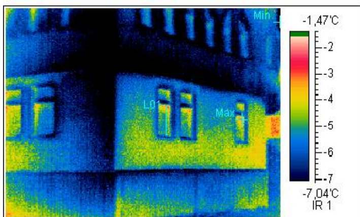
Термограмма 3
