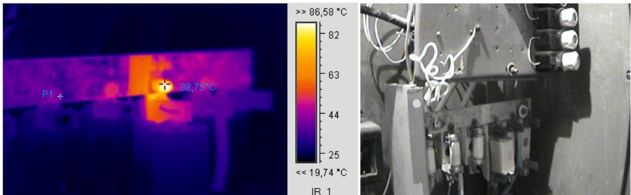
Термограмма 1
