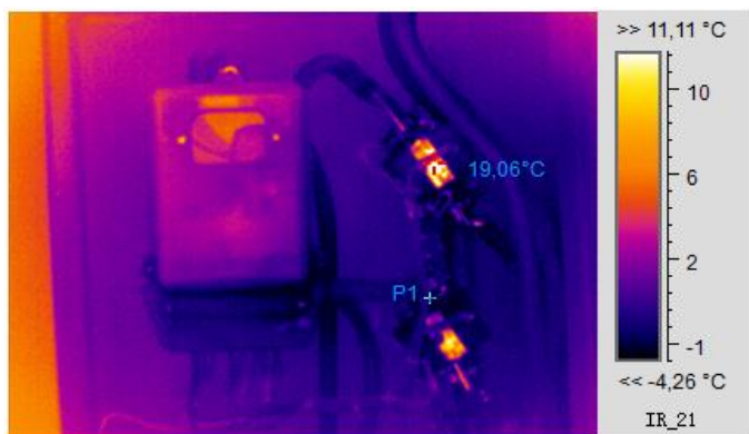
Термограмма 2
