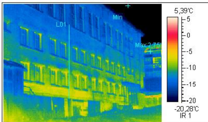
Термограмма 1
