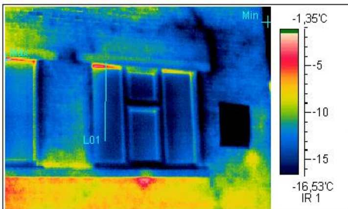
Термограмма 7
