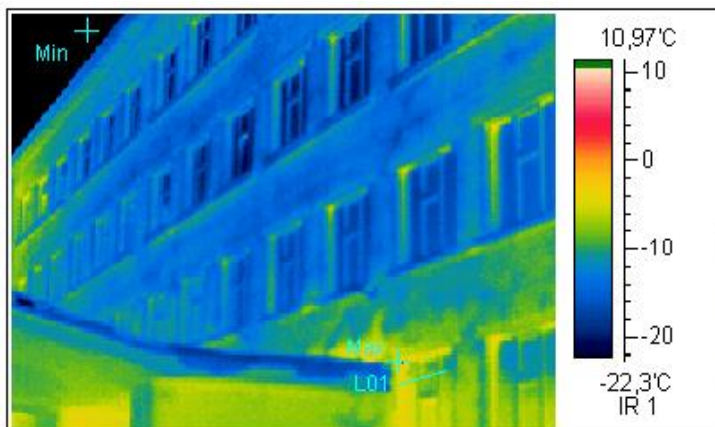
Термограмма 5
