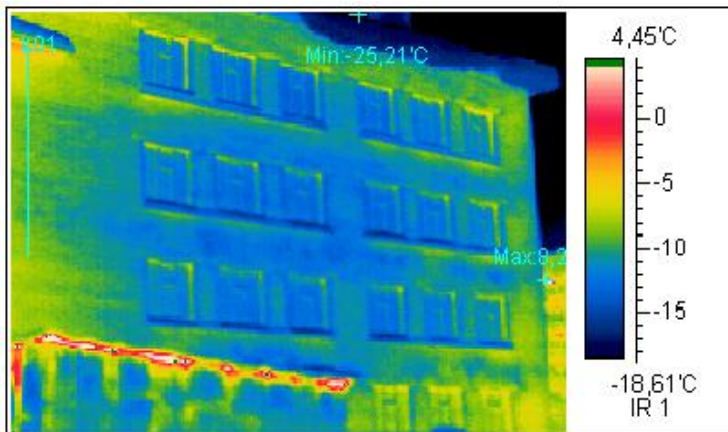
Термограмма 8
