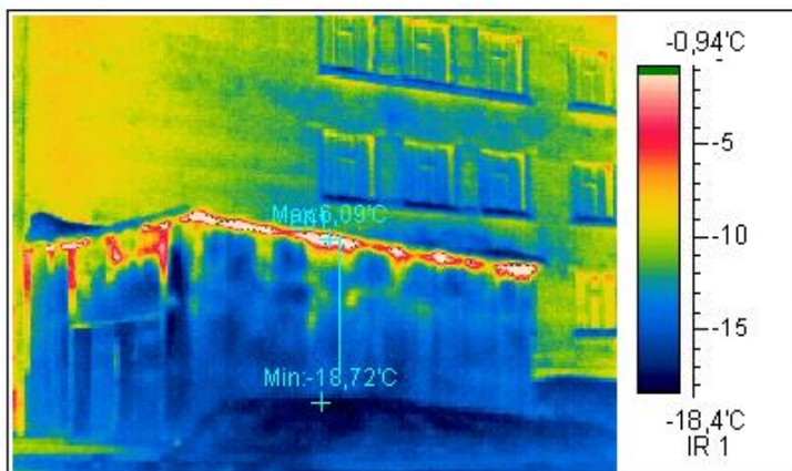
Термограмма 9
